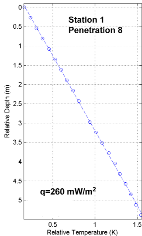
Abbildung 2: Höchster gemessener Temperaturgradient am nördlichen Rand von North Pond. Schon in 5m Tiefe liegt die Temperatur ca. 1.5°C über der Temperatur des Bodenwassers.
