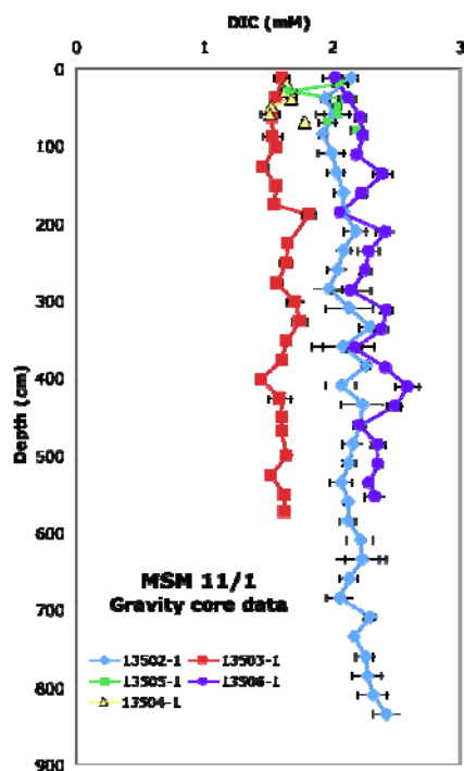
Abbildung 1: Gelöster inorganischer Kohlenstoff im Porenwasser der Schwerelotkerne. Kerne aus dem westlichen Teil von North Pond sind in blau während die anderen Kerne vom nordöstlichen Rand stammen.
